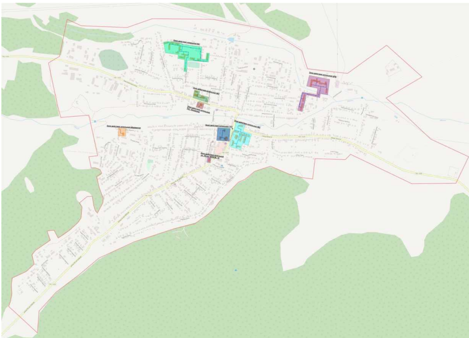
Рис. 14 - Зона действия котельных р.п. Павловка
